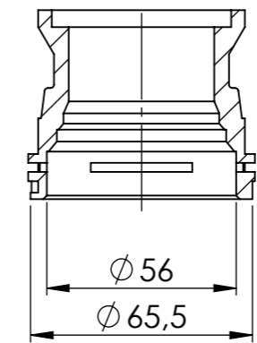
A Girişi Kesiti
