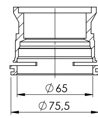
B Girişi Kesiti
