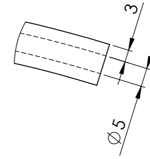
4. ve 5. Girişin Kesiti
