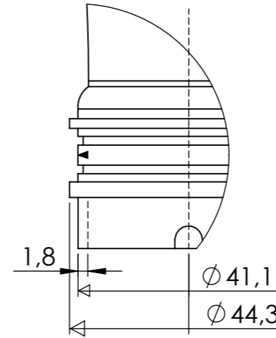
DETAY A ÖLÇEK 1 : 1
